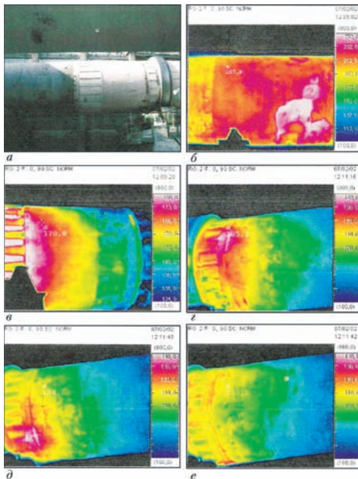
Рис. 4. Цементная печь (а) и термограммы участков с разрушающейся футеровкой (б), зон повышенной температуры в местах концентрации дефектов сварных соединений (в–е)
