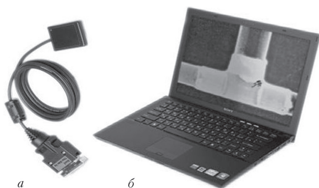
Рис. 3. Флэш-радиография с рентгеновской ПЗС матрицей фирмы «Hamamatsu Photonics»: а – ПЗС сенсор; б – рентгеновское изображение композитного тройника на экране ноутбука
