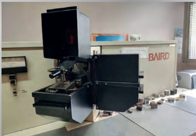
SPECTROVAC-1000 DV-4 (BAIRD, Нідерланди). Оптичний емісійний спектрометр для аналізу хімічного складу проб сплавів на залізній, нікелевій, алюмінієвій, мідній основах
