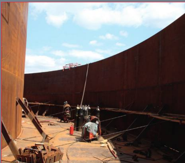
Монтаж PBC 50000
